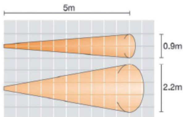
A-TL44A/B 球状ガラスレンズ 250W：最大照度70ルクス / 2.5m
