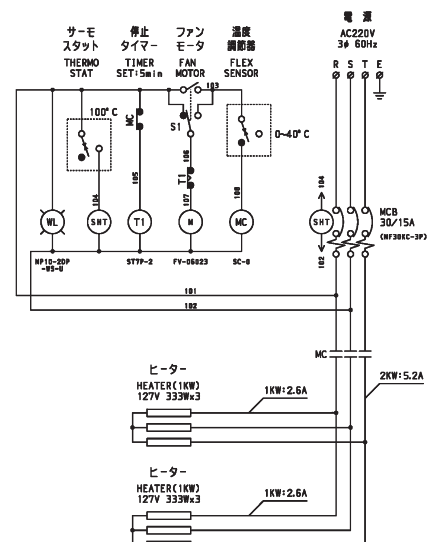
FH-322の回路例
